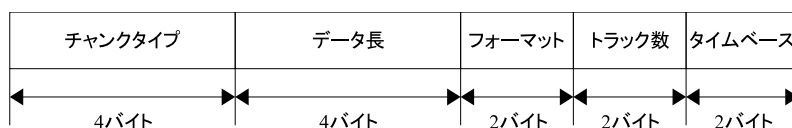
図 5.1 ヘッダチャンク
