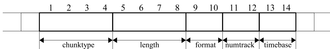
図 5.3 構造体のメモリ割り当て
