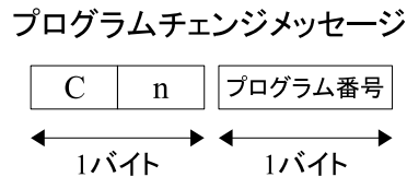
図 3.7 プログラムチェンジメッセージ
